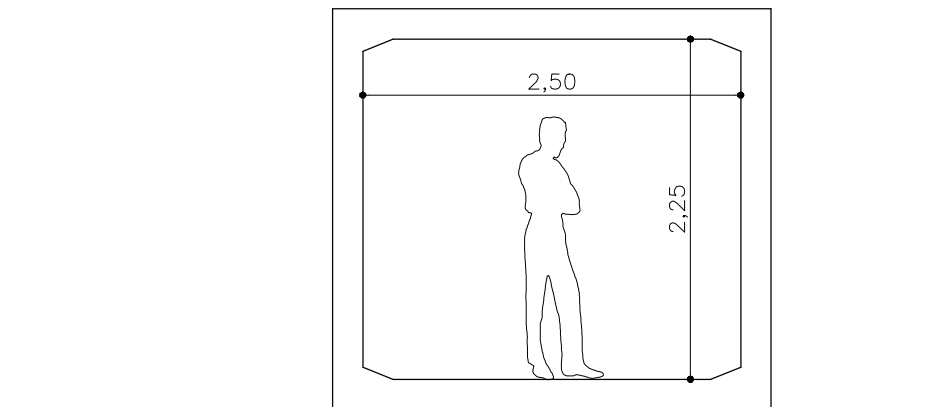
SECCIÓN
